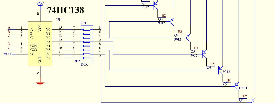
74HC138译码器实现点阵行控制
