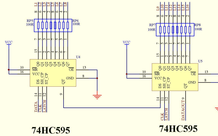
实现点阵显示列控制
